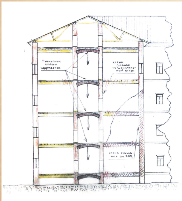
Разрез здания на Обводном канале, 19
